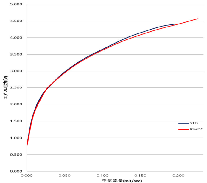
WRX STI比較フローベンチデータ
