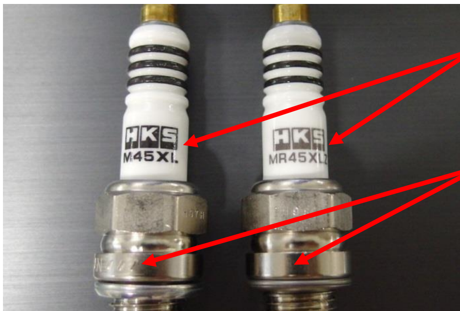
左: 変更前 右: 変更後
