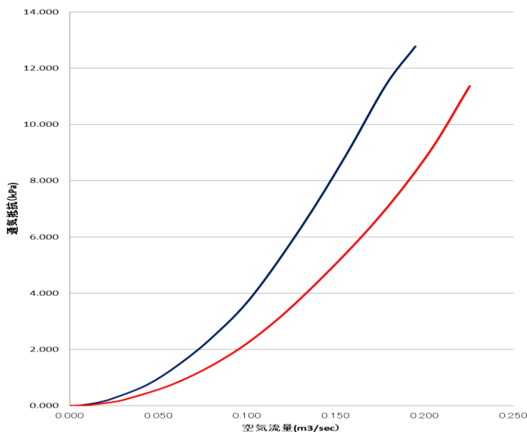
WRX STI比較フローベンチデータ
