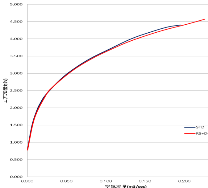
WRX STI比較フローベンチデータ
