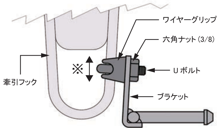
【図1.ブラケット部 詳細図】
