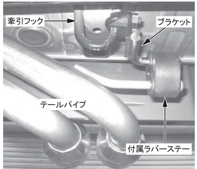
【図2.車両装着図】
