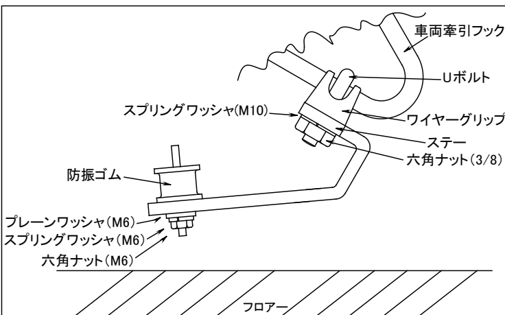
【車両側図】
