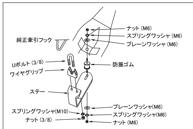
【詳細図】
