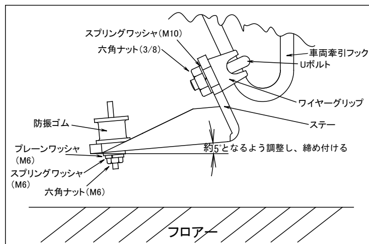
【車両側図】
