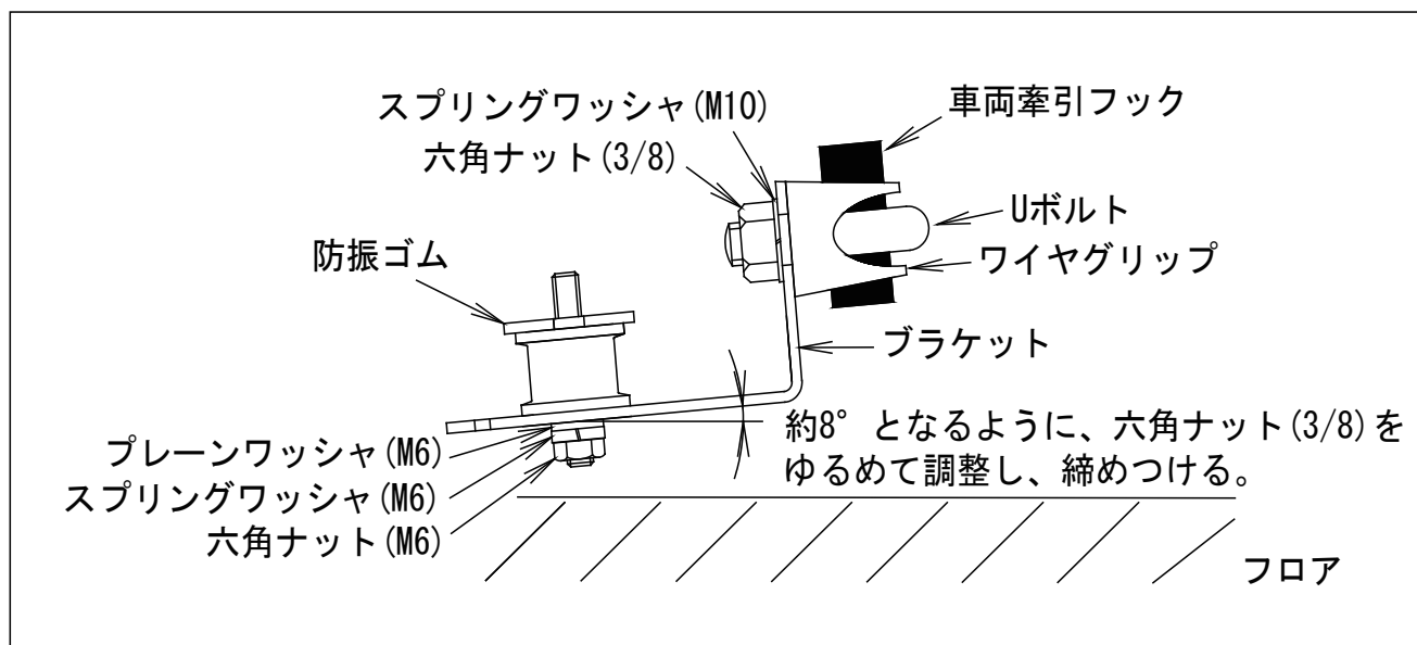
【図1.ブラケット部 詳細図】
