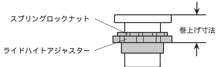
【ライドハイトアジャスター A S S Y】
