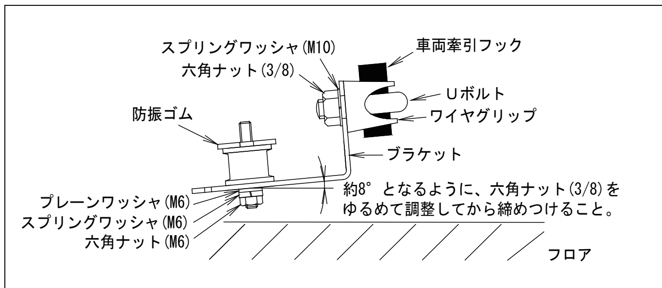
【図1.ブラケット部 詳細図】
