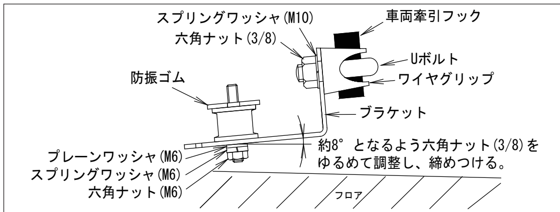
車両側ブラケット部詳細
