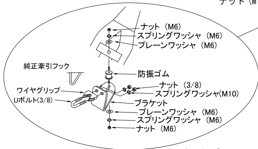
車両側ブラケット部詳細
