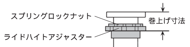
【ライドハイトアジャスター A S S Y】
