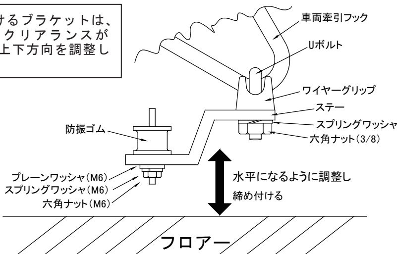
【図1.ステー部 詳細図】
