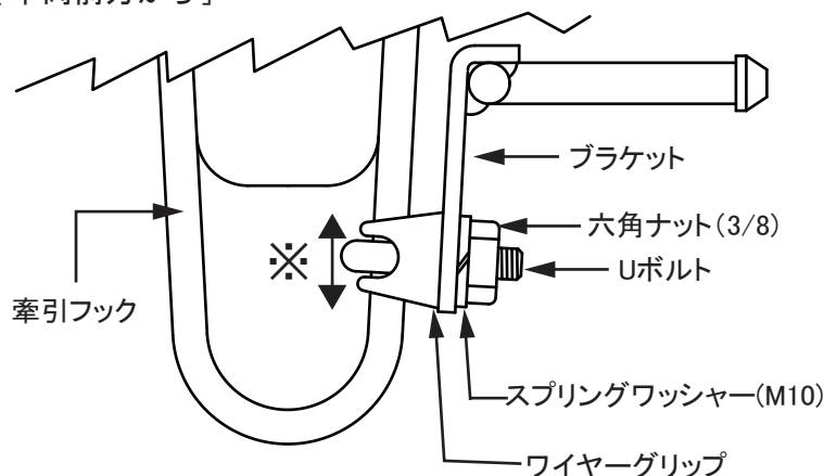
【図1.ブラケット部 詳細図】
