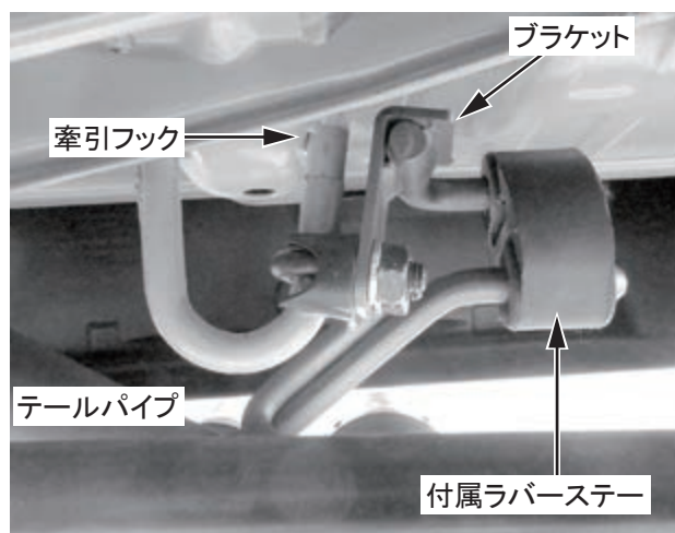
【図2.車両装着図】
