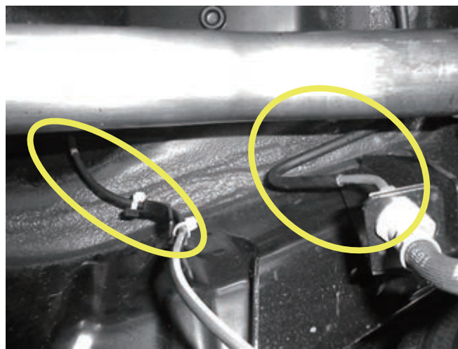
* サーマシール貼付け箇所 (拡大図)
