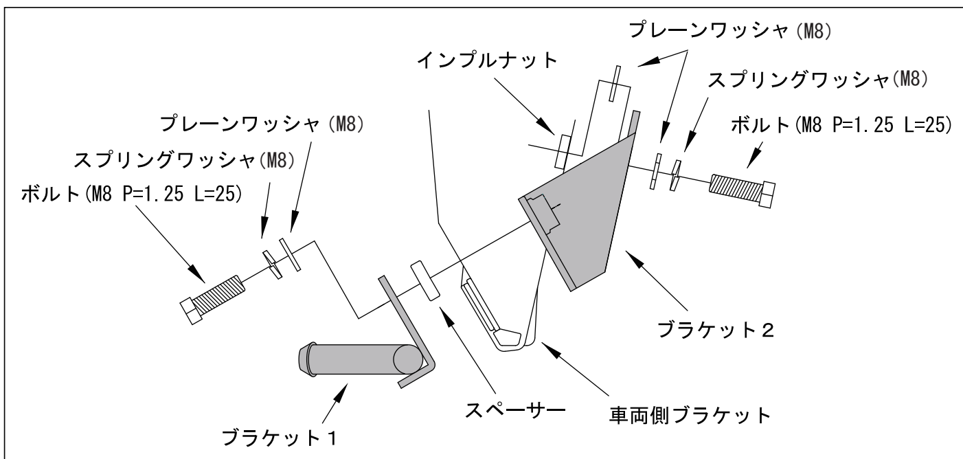
【図4.ブラケット組付詳細図】
