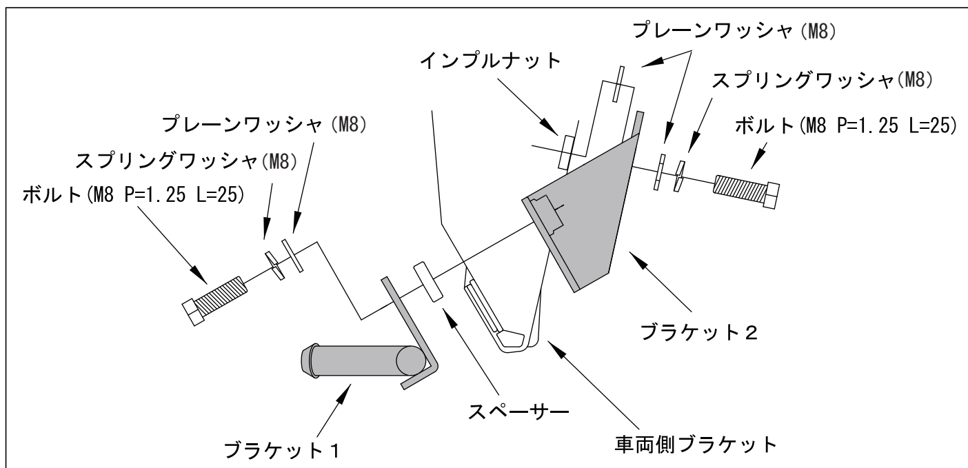
【図4.ブラケット組付詳細図】
