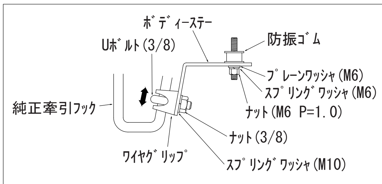
【図1.ブラケット部 詳細図】
