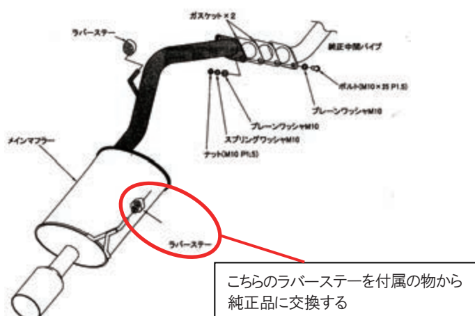
図4 メインマフラー構成図
