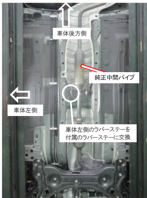
図3 交換するラバーステーの位置
