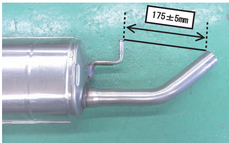
図2. 純正マフラー切断位置
