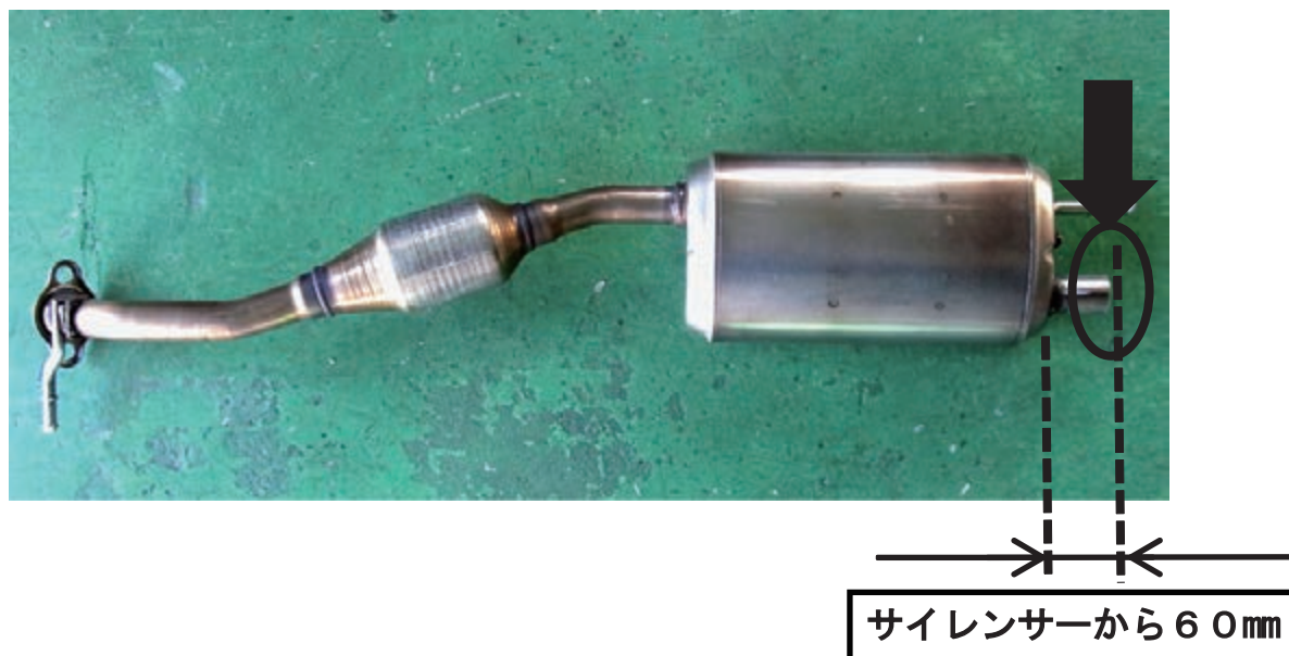
図2. 純正マフラー切断位置
