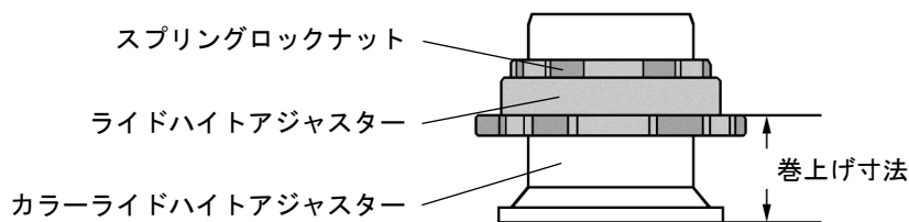
【ライドハイトアジャスターASSY】
