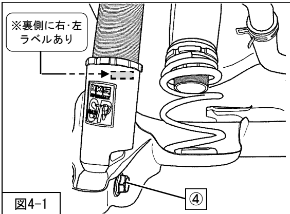
リアショックアブソーバASSY取付方向
