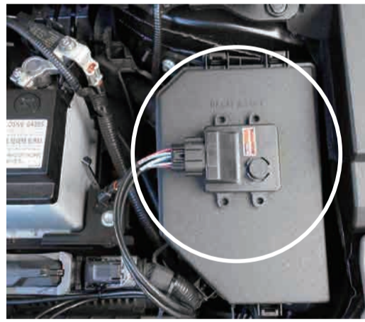
Power Editor 本体を設置・固定
