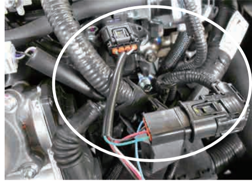
Power Editor ハーネスを割込み接続
