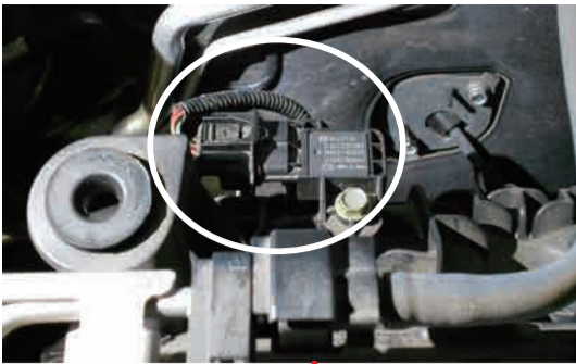
圧力センサ位置（チャンネル1側）
