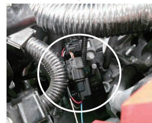
Power Editor ハーネスを割込み接続
