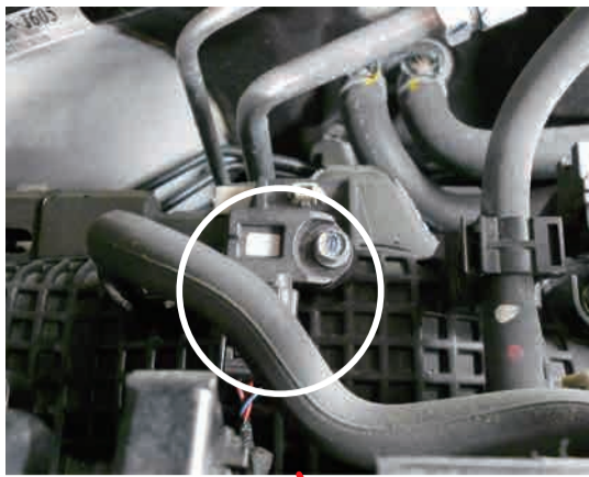
圧力センサ位置（チャンネル2側）
