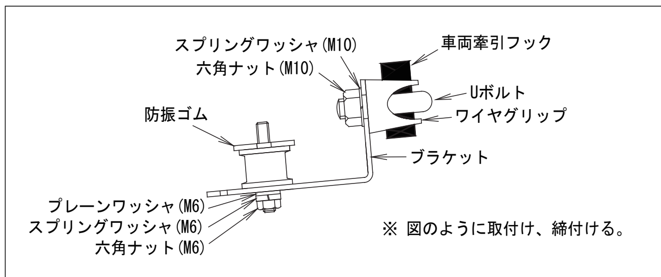
【図1.ブラケット部 詳細図】
