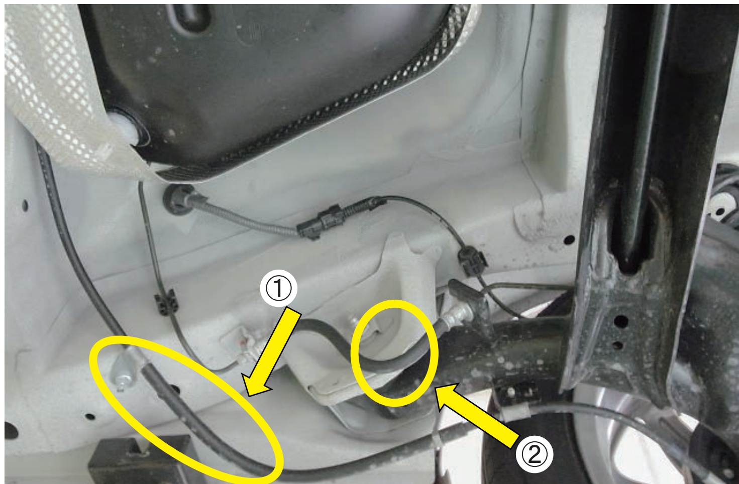
図 4. サーモシール貼付け箇所写真
