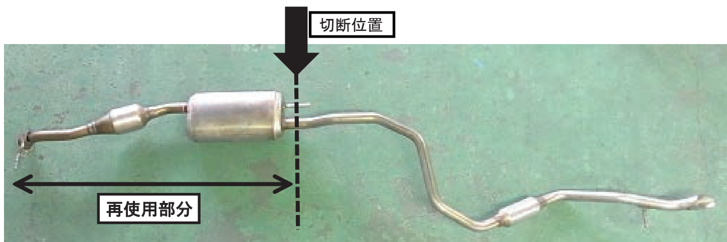
図1. 純正マフラー切断位置
