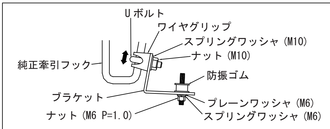
【図1.ブラケット部 詳細図】
