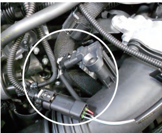
Power Editor ハーネスを割込み接続
