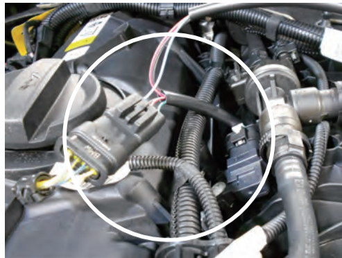
Power Editor ハーネスを割込み接続
