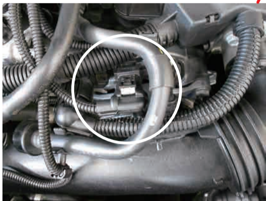
圧力センサ位置（チャンネル2側）
