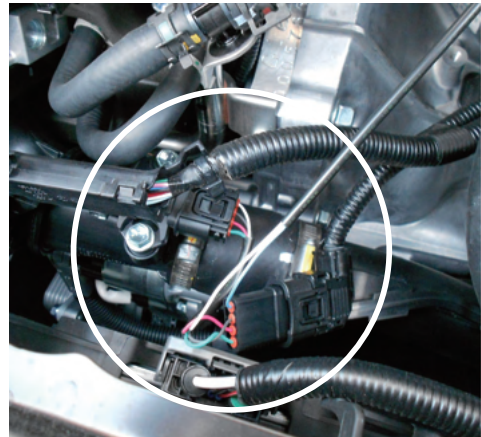
Power Editor の接続ハーネスを割込み接続
