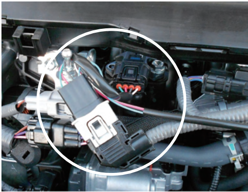
Power Editor の接続ハーネスを割込み接続
