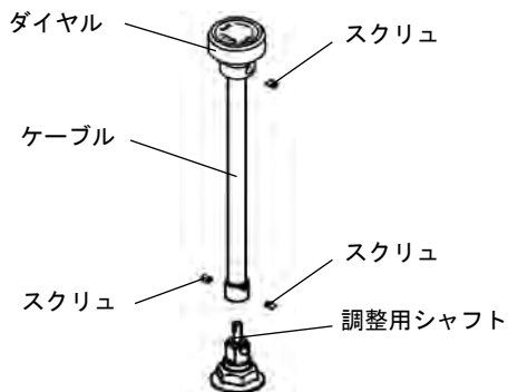
図4-6 : NA6CE・NA8C 左側
