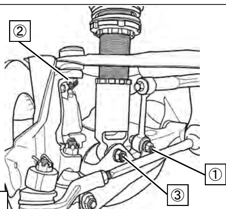
図2-3 : ABS装着車
