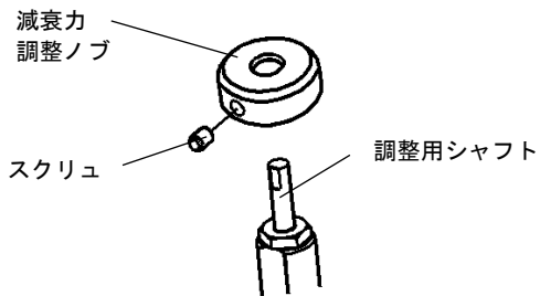
図4-5 : NA6CE・NA8C 右側
