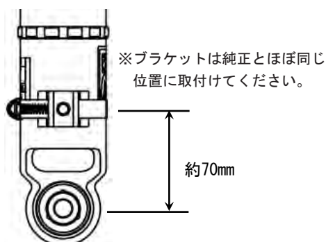
図2-1 : ABS装着車
