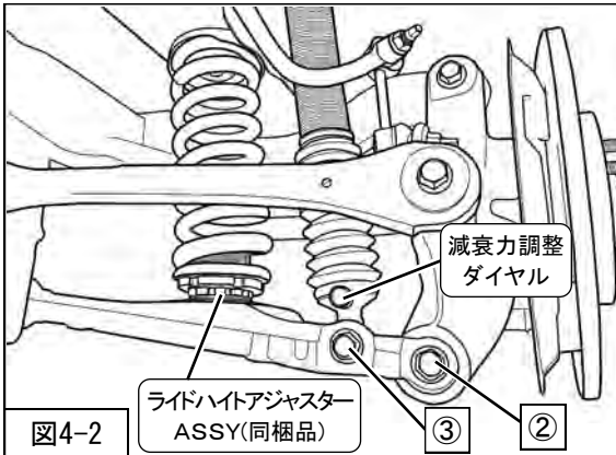
リアショックアブソーバASSY
