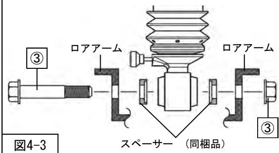
リアショックアブソーバASSY
