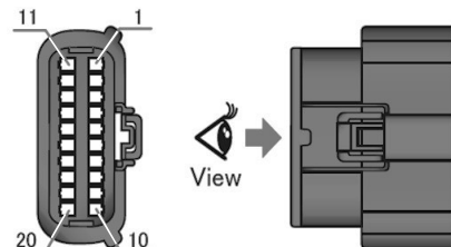
Power Editor R 本体側コネクタ
